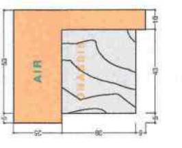
ΟΨΗ 13 ΚΑ. 1:25
